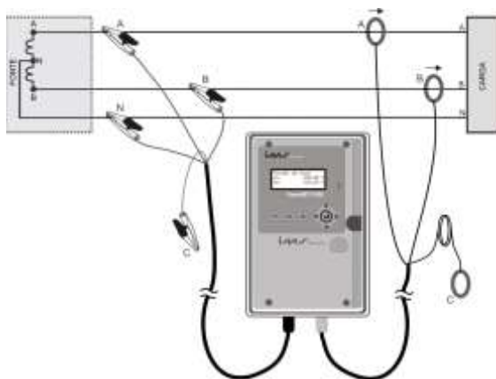
Sistema 03: 2P3W-2V2C - Bifásico (LL+LN)
